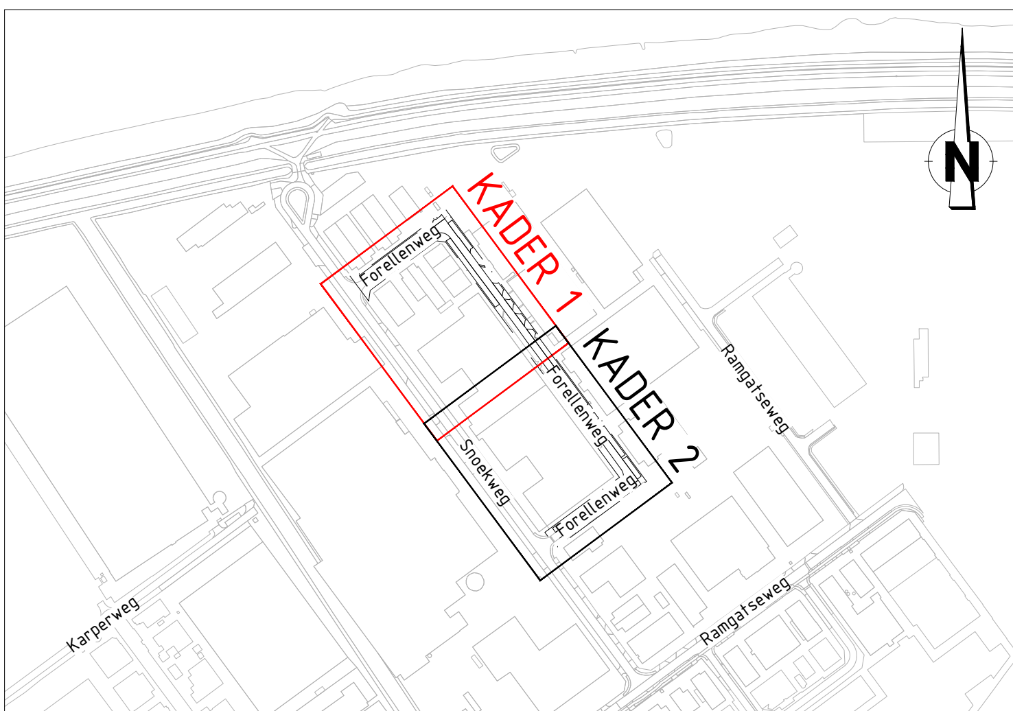
Situatieoverzicht SCHAAL 1 : 5.000
