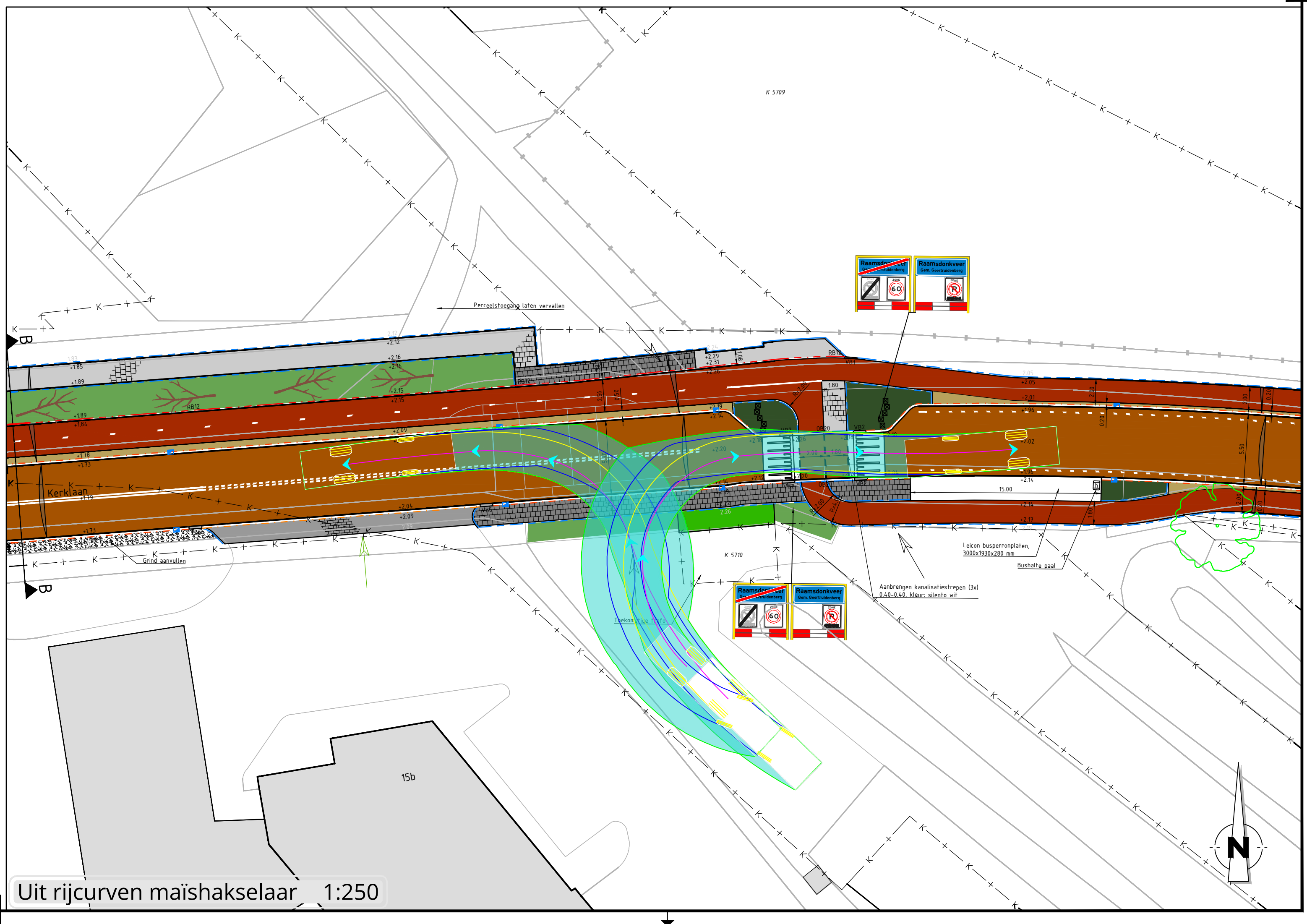
Uit rijcurven maishakselaar 1:250
