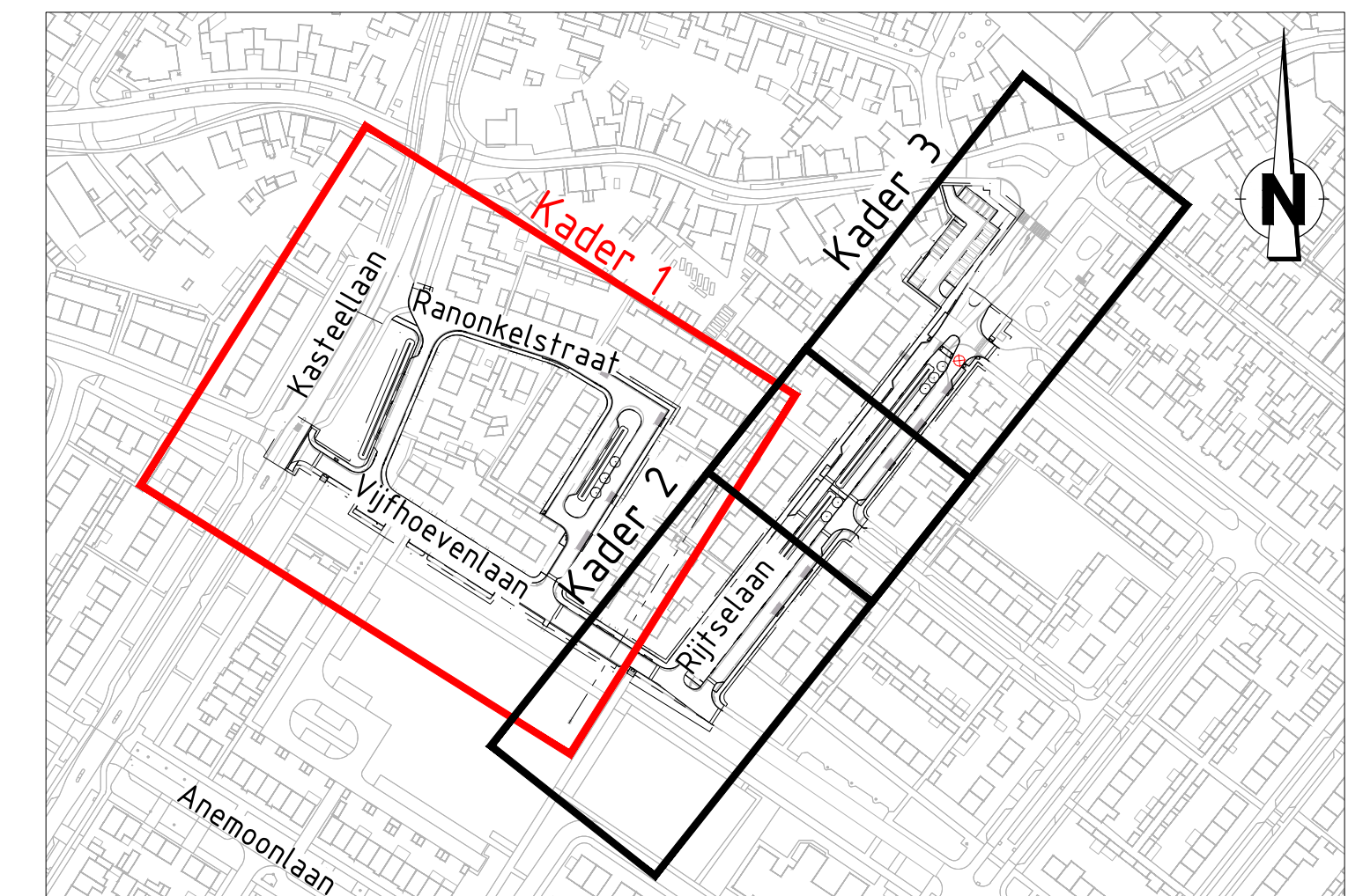
Situatieoverzicht SCHAAL 1 : 2500
